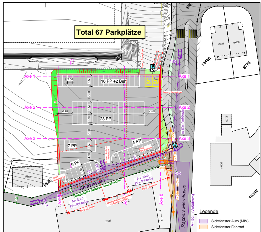
Situationsplan Churzhaslen 1:500 (weitere Pläne auf www.eschenbach.ch )
