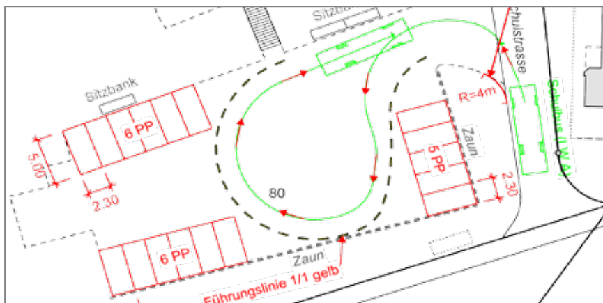
Situationsplan Schulhausplatz St. Gallenkappel
